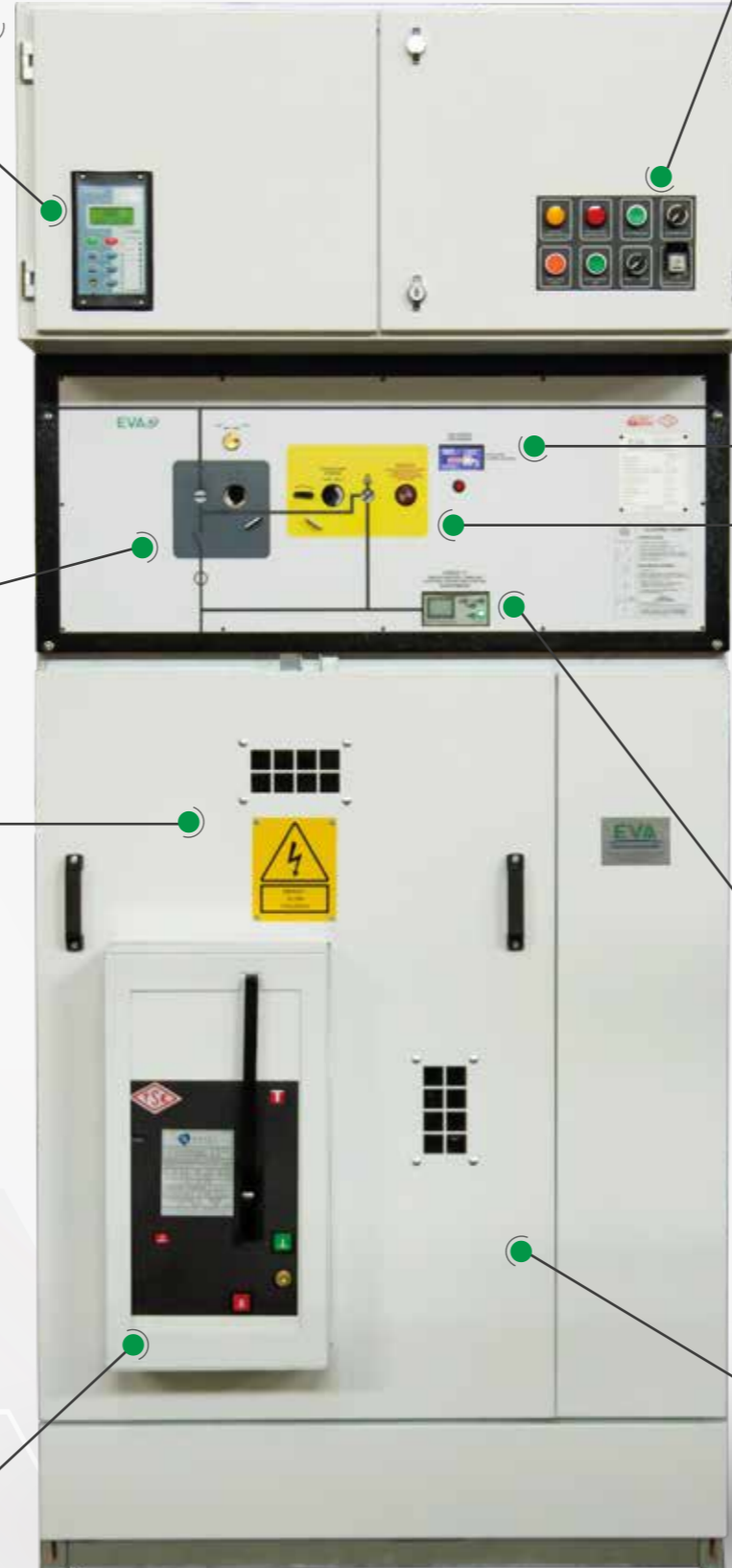
Kontaklı gerilim gösterge indikatörü sayesinde hücrenin enerjili olup olmadığını scada sisteminden takip edebilme imkanı.
